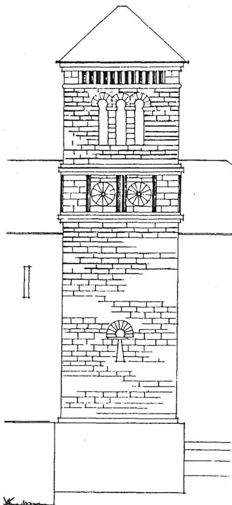
Alzado Sur
